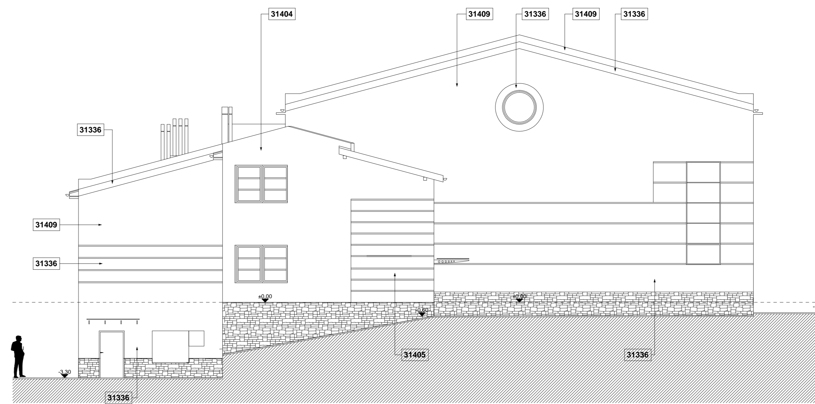
ELEWACJA PÓŁNOCNA
